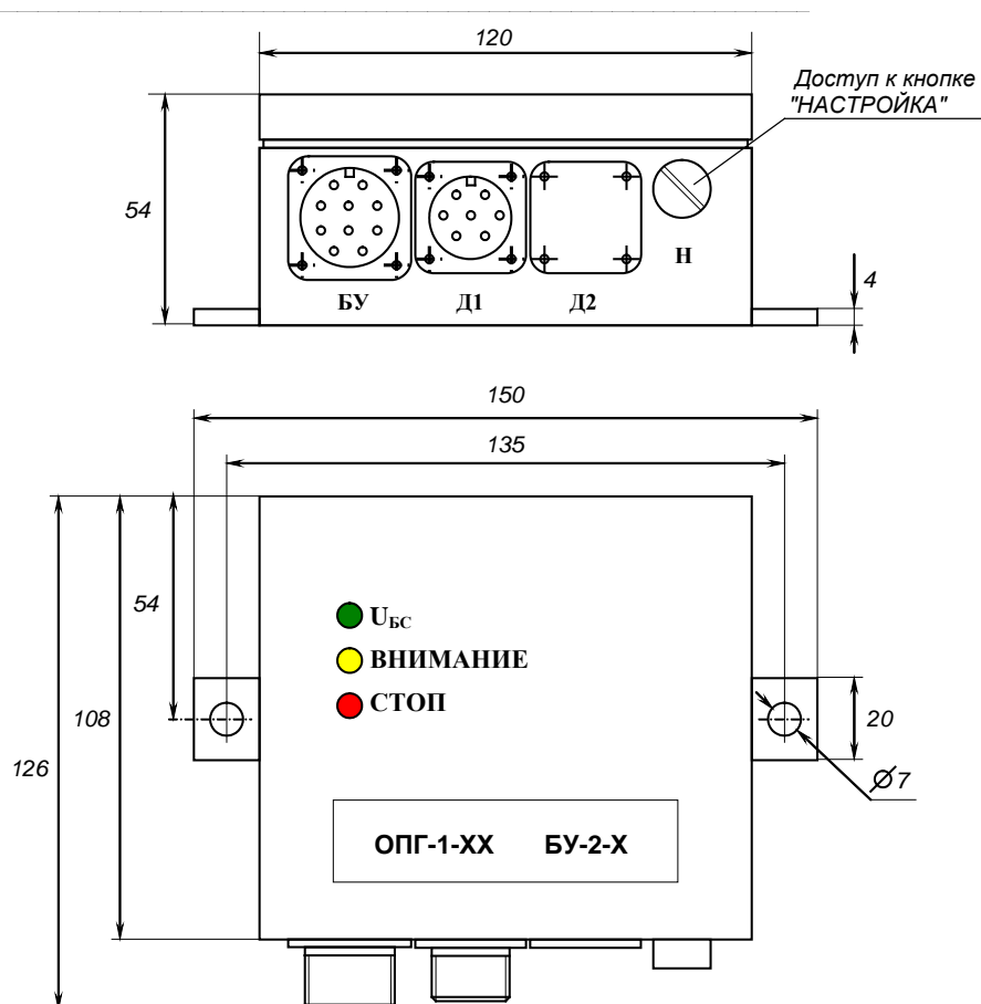
Рисунок 5 – Габаритные и присоединительные размеры БУ-2
