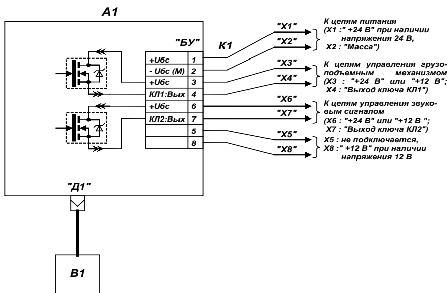
A1 – Блок управления БУ-2-4 В1 – Преобразователь давления (ПрД) К1 – Жгут ЛГФИ.685625.046
