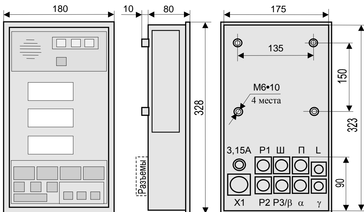
Рисунок 7 - Габаритные и присоединительные размеры БОДа
