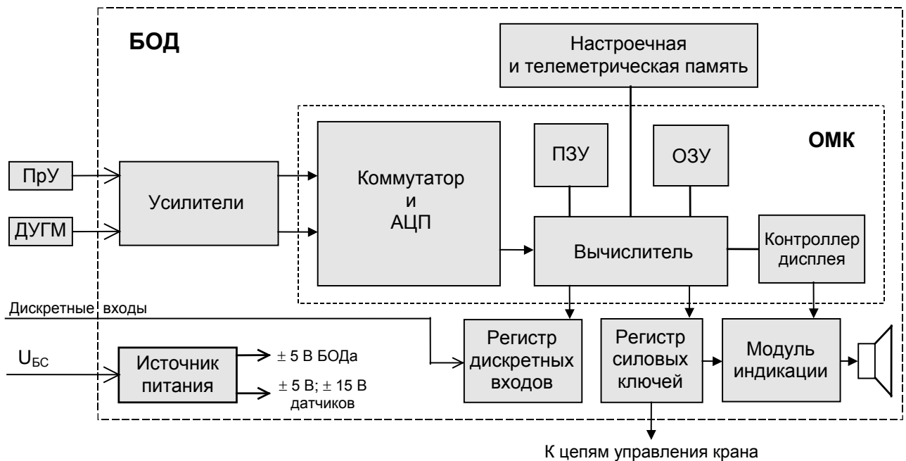
Рисунок 1 - Блок-схема ограничителя
