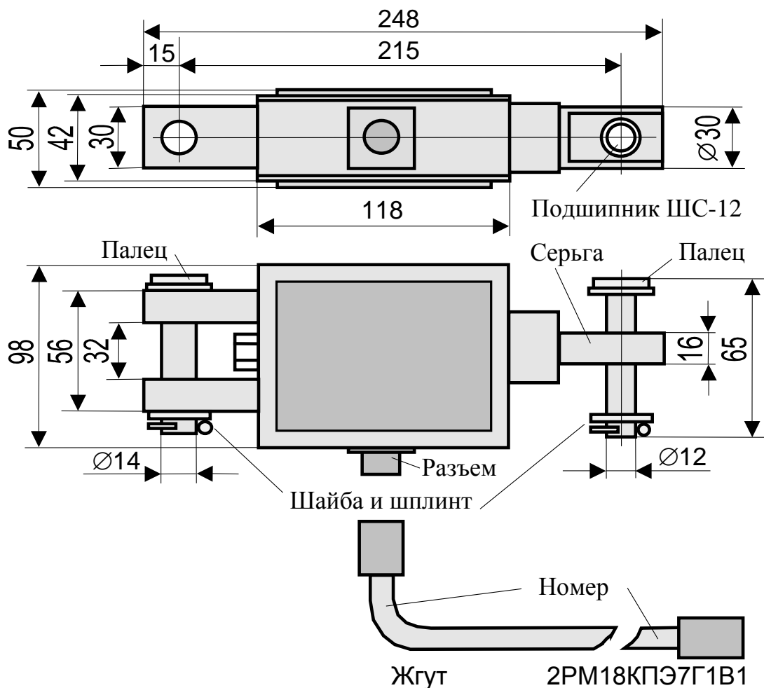
Рисунок 5 - Преобразователь усилия
