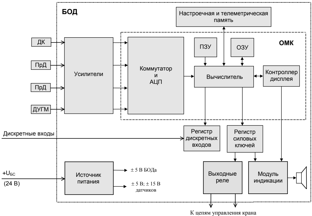
Рисунок 1- Блок-схема ограничителя
