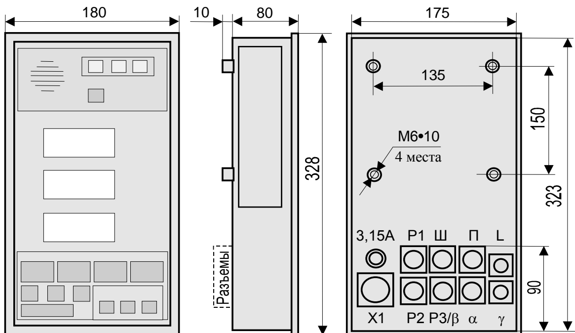
Рисунок 5 - Габаритные и присоединительные размеры БОД
