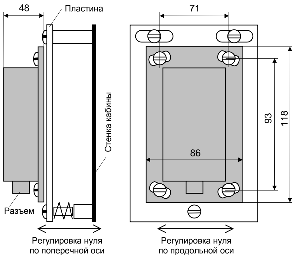
Рисунок 8 - Установка датчика крена
