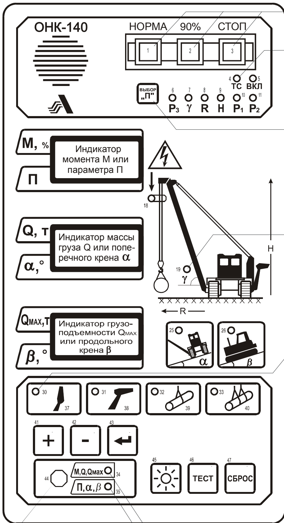
Рисунок 4 - Лицевая панель ограничителя ОНК-140-72
