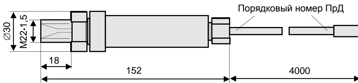
Рисунок 6 - Преобразователь давления
