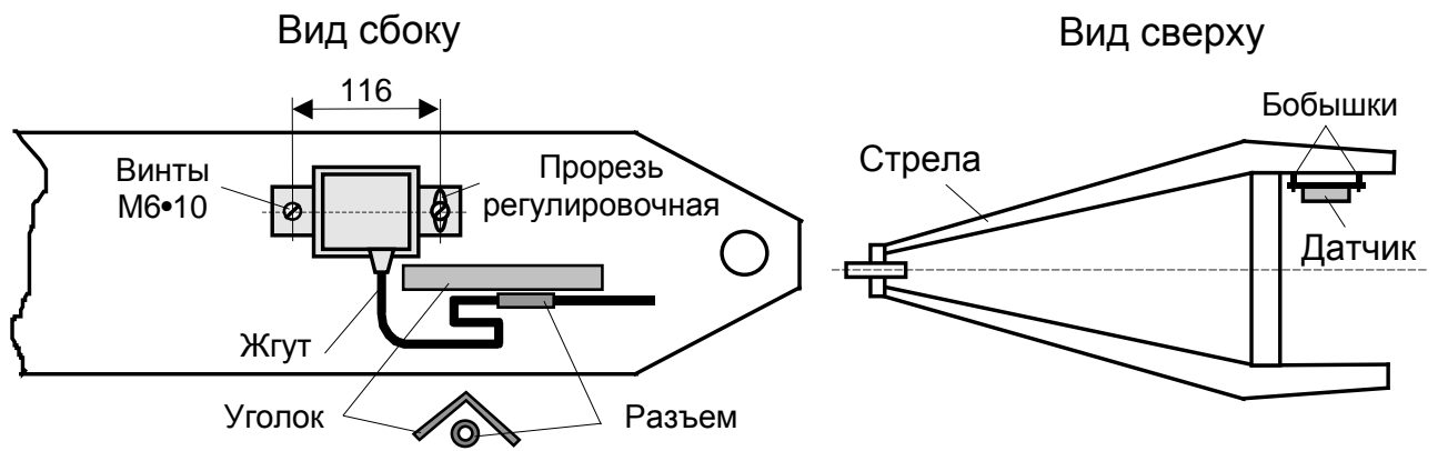
Рисунок 7 - Установка датчика угла маятникового
