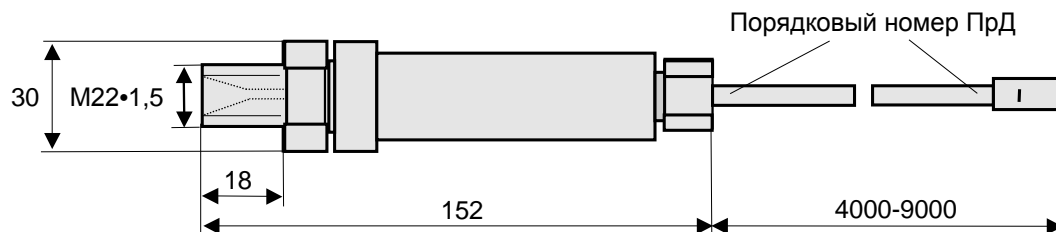
Рисунок 8 - Преобразователь давления
