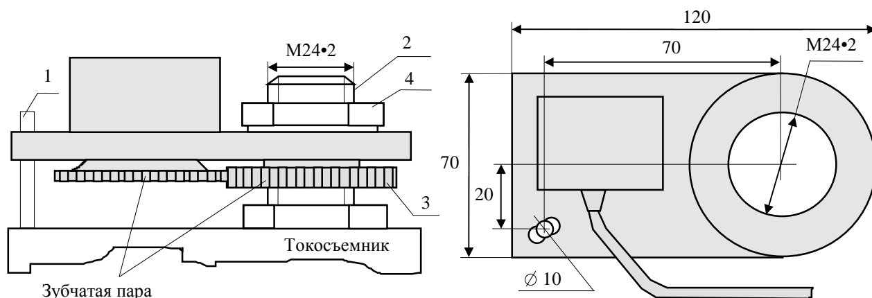
Рисунок 6 - Установка датчика азимута
