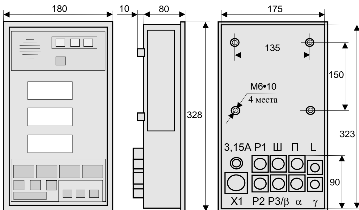
Рисунок 10 - Габаритные и присоединительные размеры БОДа
