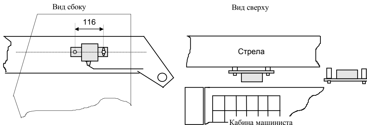
Рисунок 5 - Установка датчика угла маятникового
