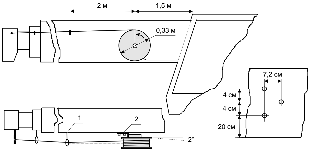
Рисунок 9 - Установка датчика длины стрелы и разметка мест крепления
