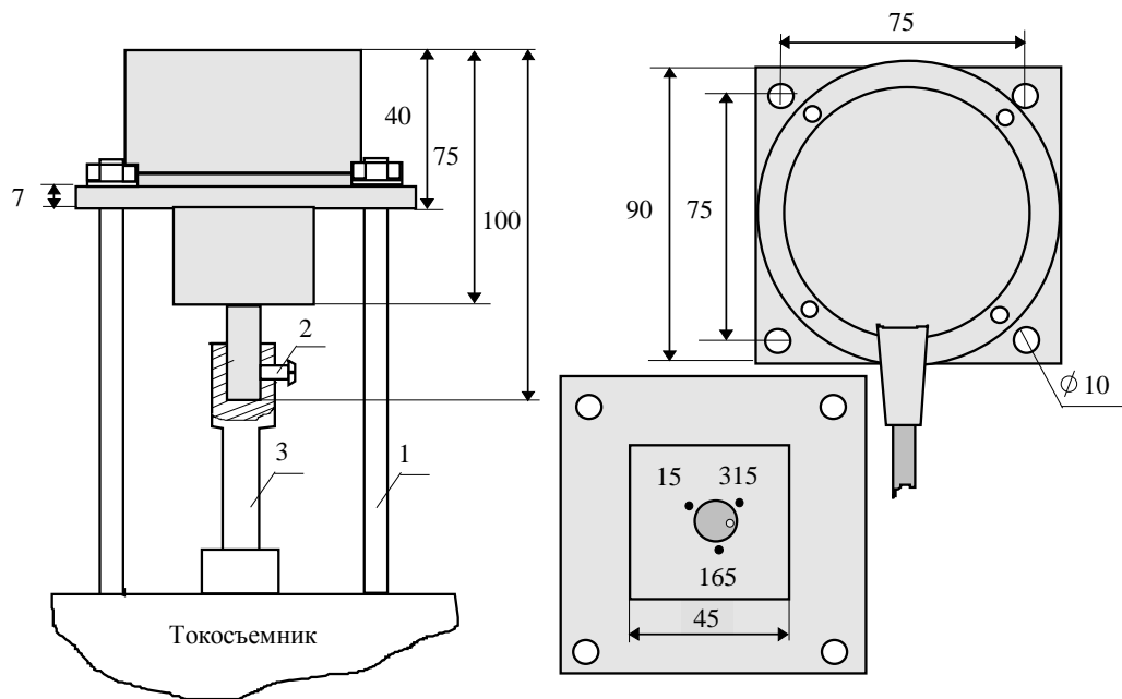
Рисунок 7 - Установка датчика угла
