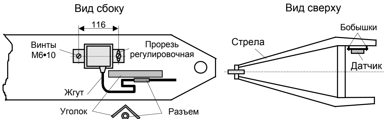
Рисунок 5 - Установка датчика угла маятникового
