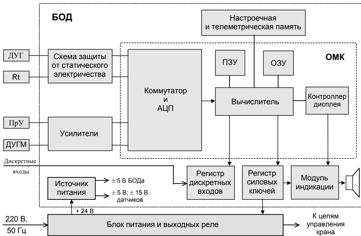
Рисунок 1 - Блок-схема ограничителя
