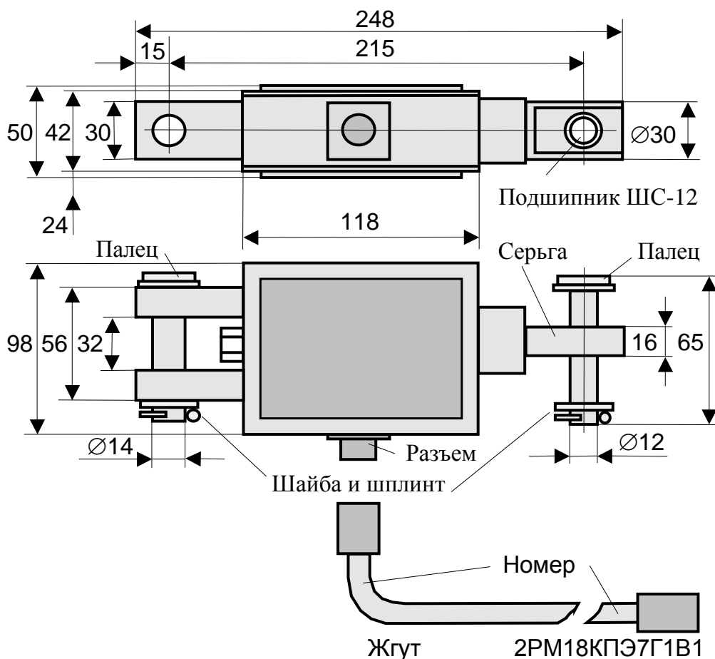
Рисунок 7 - Преобразователь усилия
