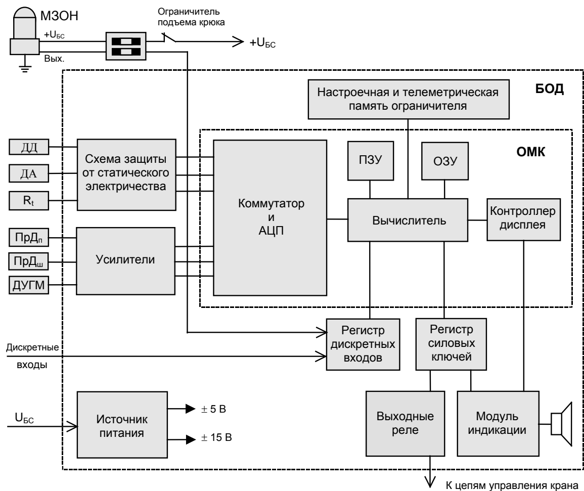
Рисунок 1- Блок-схема ограничителя
