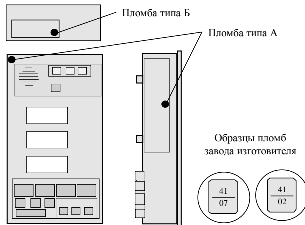
Рисунок 3 - Расположение пломб на БОДе
