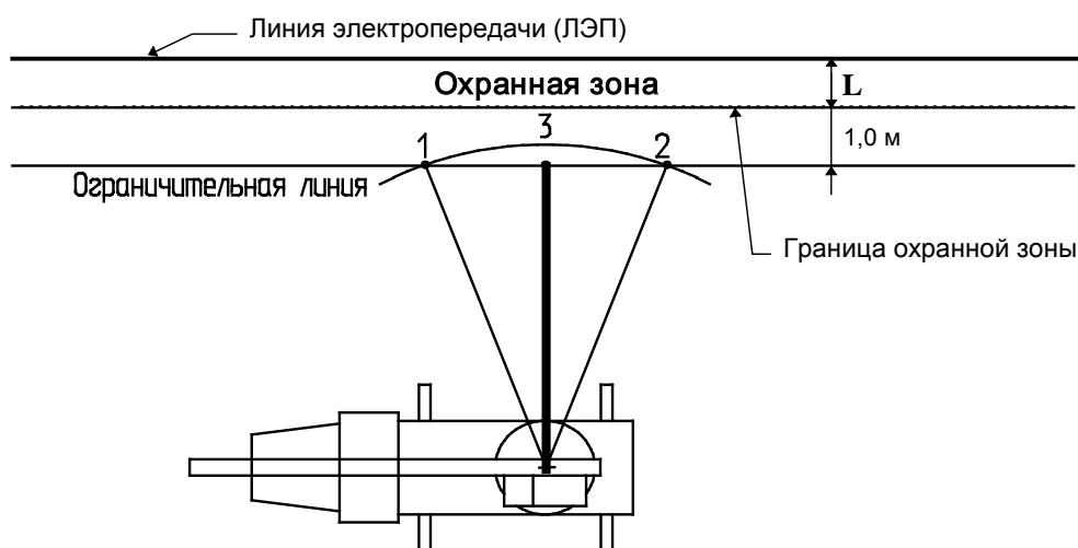
Рисунок 5 - Ввод ограничения "Стена"
