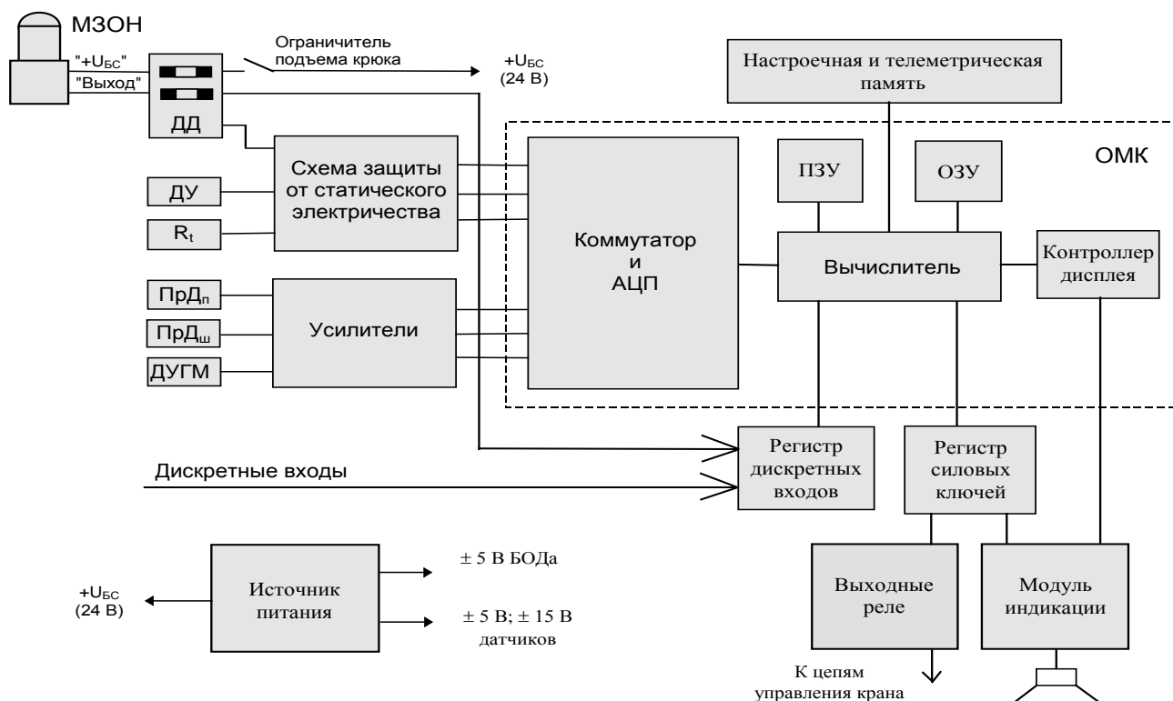
Рисунок 1 - Блок-схема ограничителя
