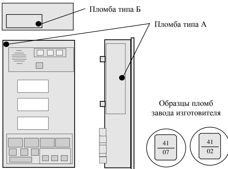
Рисунок 3 - Расположение пломб на БОДе
