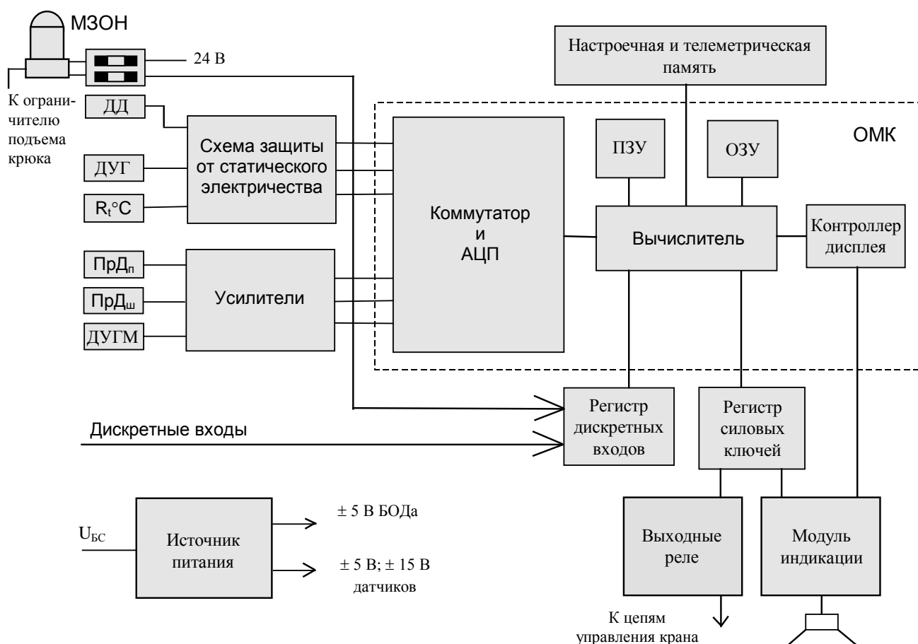
Рисунок 1- Блок-схема ограничителя
