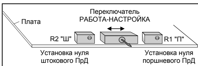
Рисунок 7 – Размещение регулировочных резисторов на плате БОДа
