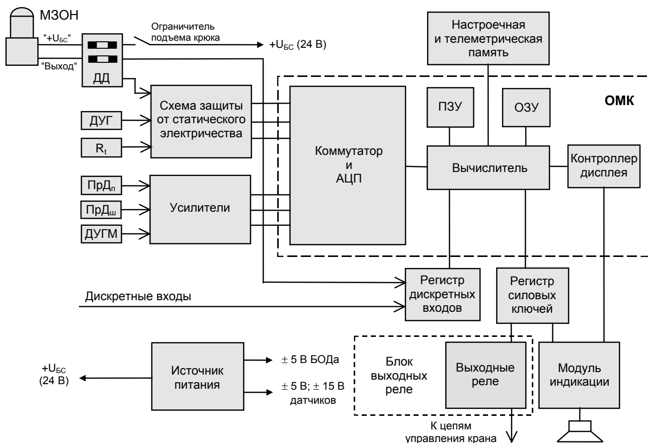
Рисунок 1- Блок-схема ограничителя
