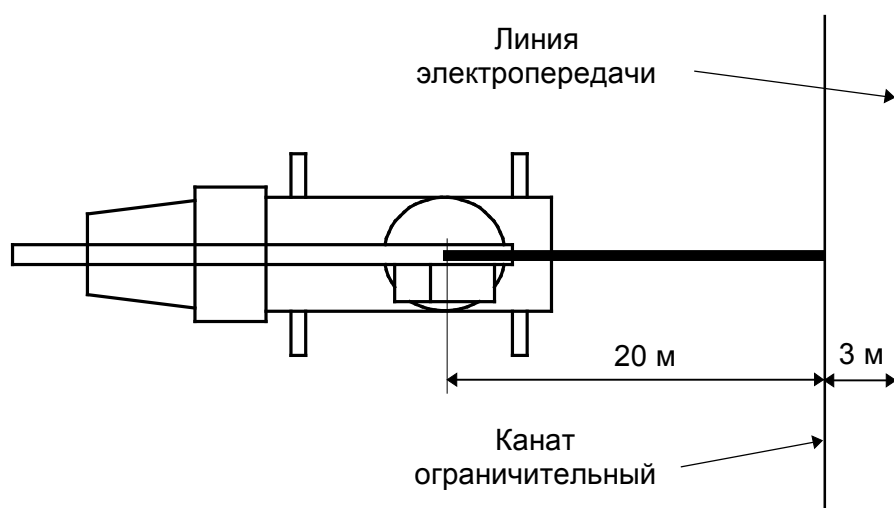
Рисунок 6 - Проверка срабатывания МЗОНа
