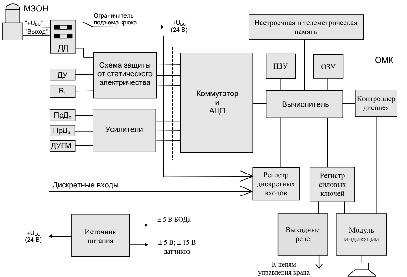
Рисунок 1- Блок-схема ограничителя
